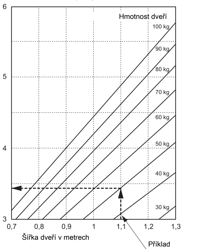
Minimální doba otevírání/zavírání křídlových dveří, čas t pro vyhovění LE
